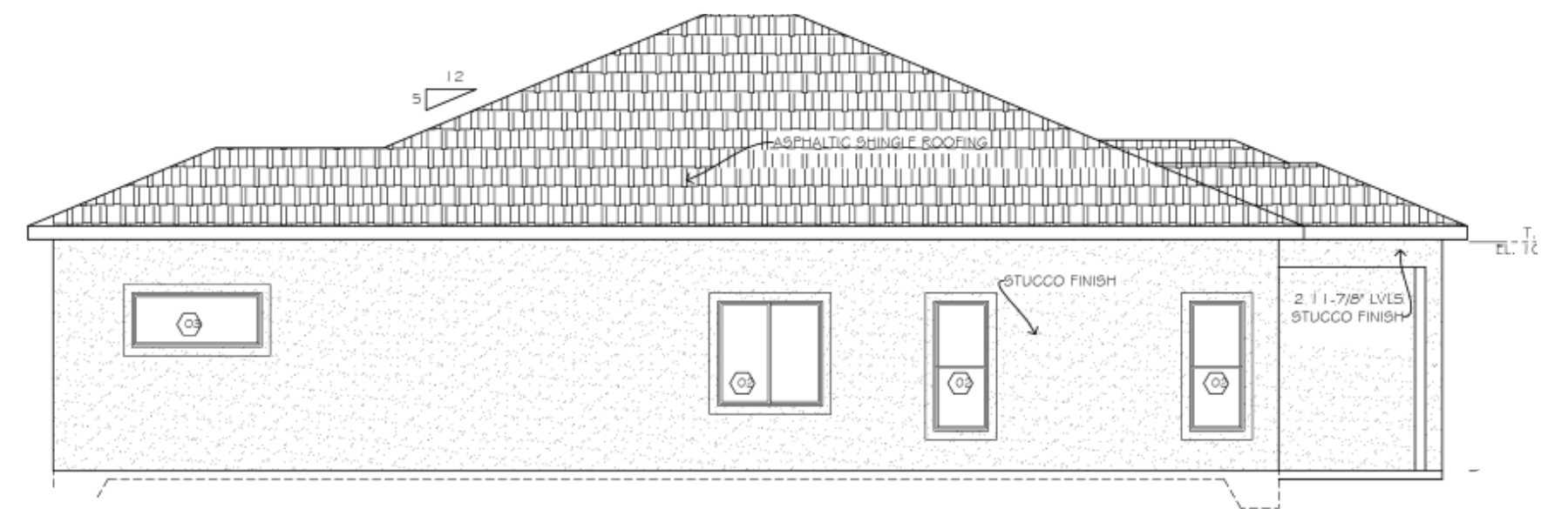
Right Elevation
